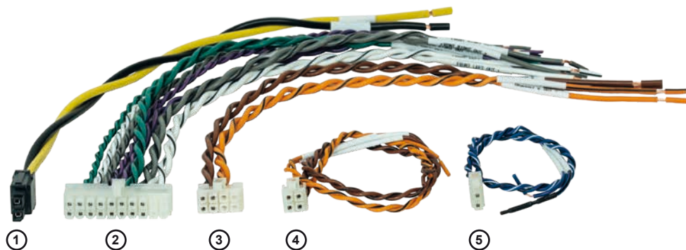
Abb. 2: Übersicht Anschlusskabel
