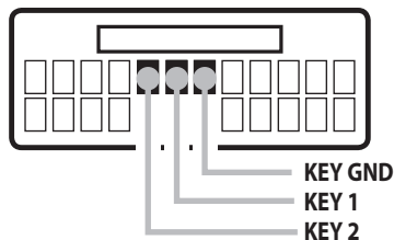
DIAGRAMA DE CONEXIONES VM001
